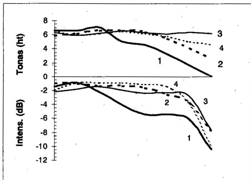
2 pav. Priegaidės kirčiuotuose dvigarsiniuose skiemenyse (1 – SK akūtas, 2 – JK akūtas, 3 – SK cirkumfleksas, 4 – JK cirkumfleksas)
