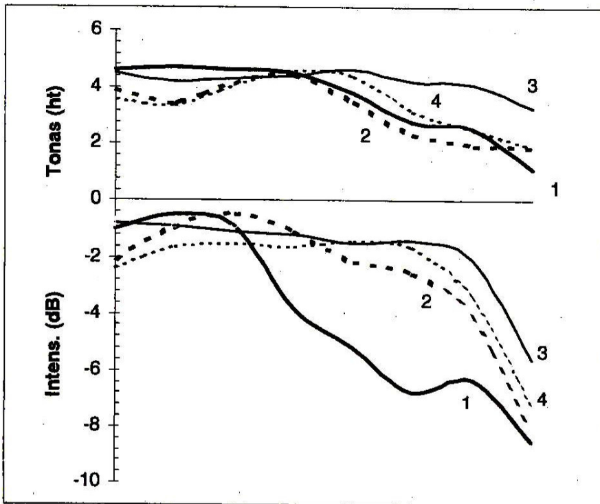
1 pav. Pagrindinio kirčio priegaidės vienabalsiniuose skiemyse (1 – SK akūtas, 2 – JK akūtas, 3 – SK cirkumfleksas, 4 – JK cirkumfleksas)
