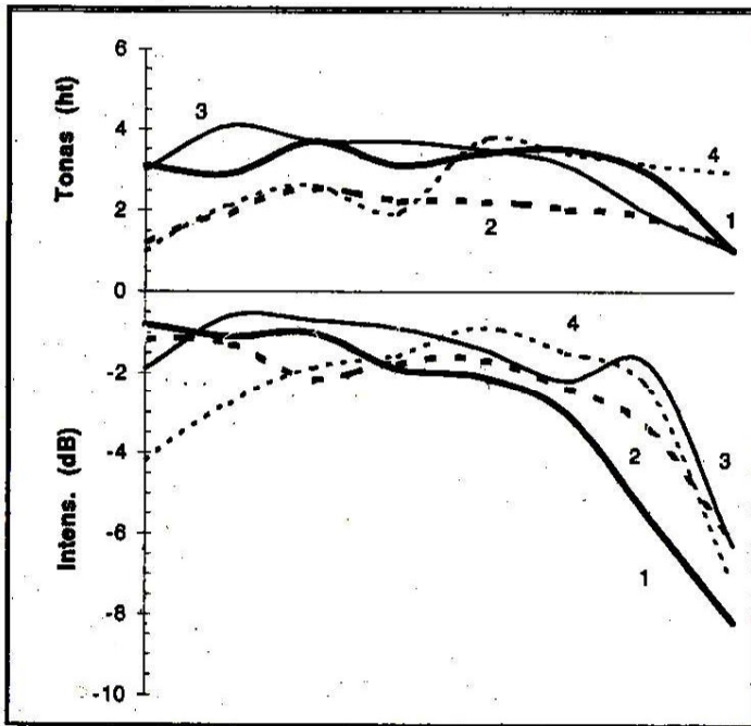
3 p a v. Atitrauktinio kirčio priegaidės dvigarsiniuose skiemenyse (1 – SK „akūtas“, 2 – JK „akūtas“, 3 – SK „circumflexas“, 4 – JK „circumflexas“)
